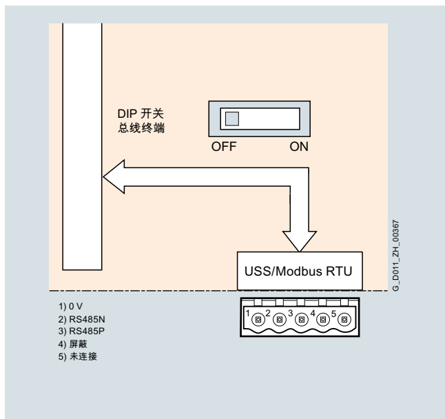
USS/Modbus RTU 通讯接口
