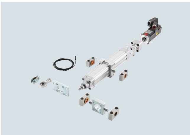
SIMOTICS S-1FK7 电机轴向安装在直线单元上，含安装套件及附件
