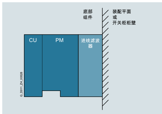
由功率模块 (PM) 和控制单元 (CU) 以及作为底部组件的进线滤波器构成的变频器 (侧视图)
