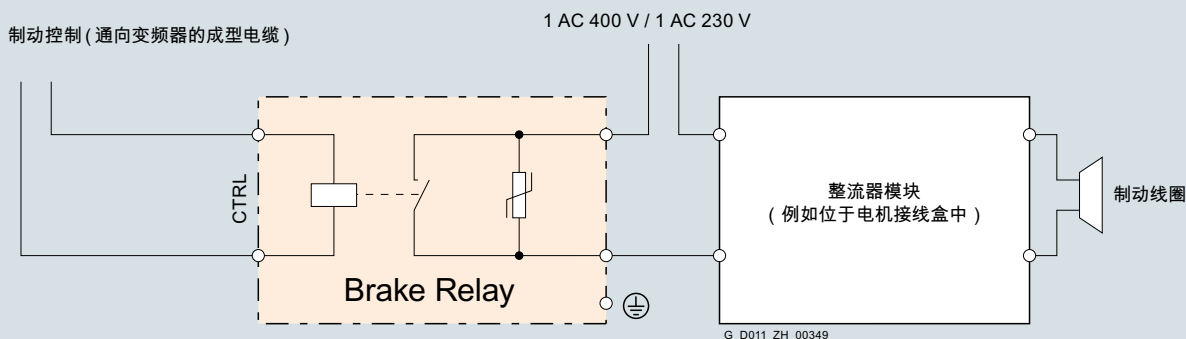
制动继电器的连接示例，1 AC 230 ... 400 V
