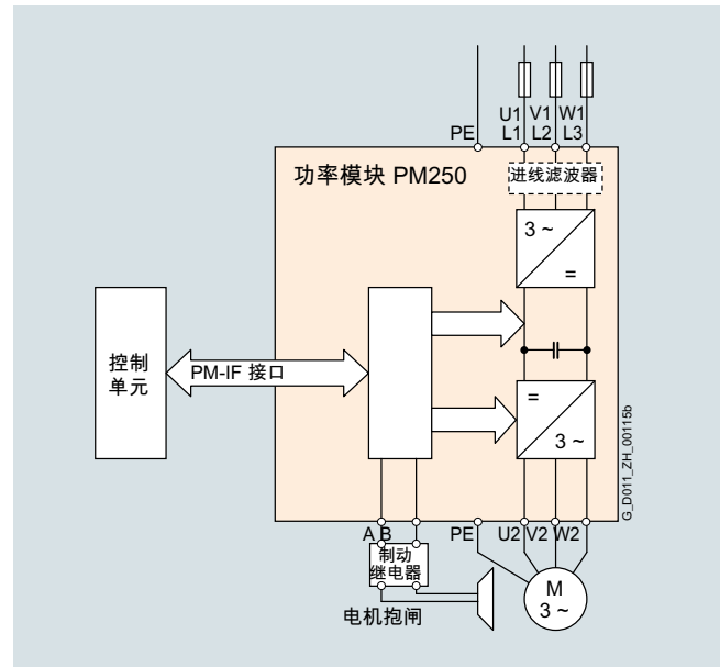
集成或未集成进线滤波器的功率模块 PM250 的接线示例
