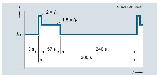
基于高过载的负载循环 300 s
