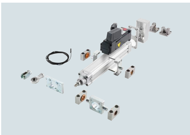
SIMOTICS S-1FK7 电机平行安装在直线单元上，含安装套件及附件
